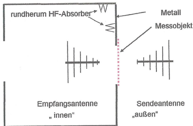
Bild 1: Messanordnung nach IEEE 299-2006 zur Bestimmung der Schirmdämpfung
